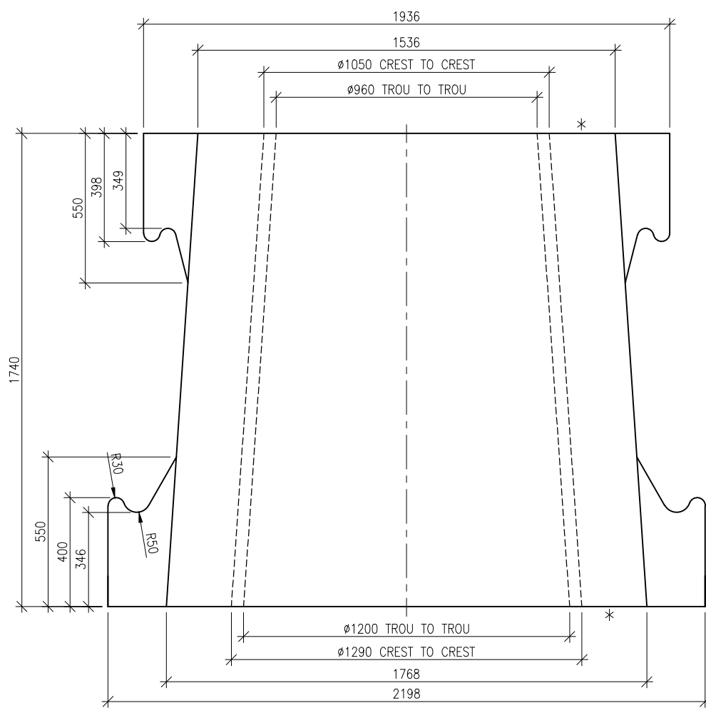
ELEVATION
